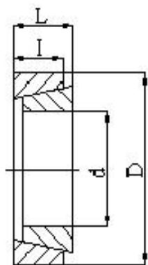
Z1型胀紧联接套的基本尺寸及参数
