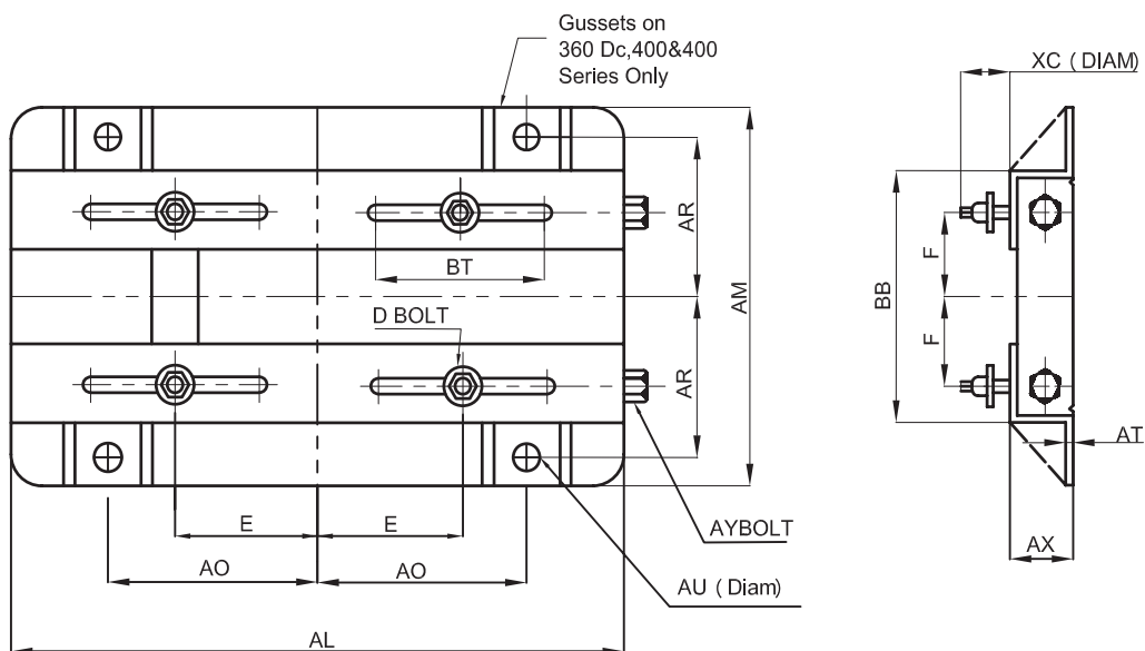
MB型电机底座的基本参数和尺寸
